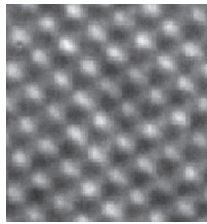
シリコン単結晶（(110)面）の高分解能TEM像
